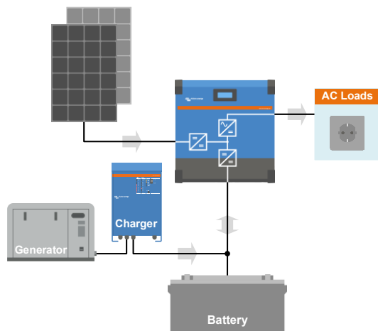
Exemple de système avec générateur Ajouter un générateur et un chargeur de batterie si davantage de puissance est nécessaire.
